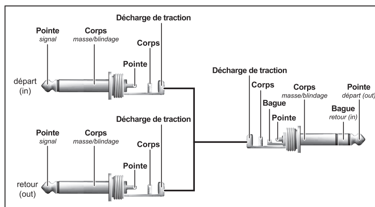
Fig. 5.1 : Câble d'insert avec deux jacks mono et un jack stéréo
