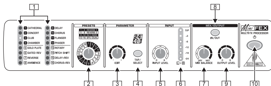
Fig. 2.1 : Commandes de la face avant du FEX800
