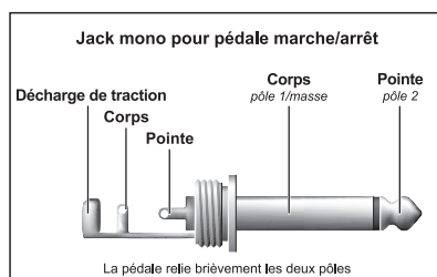
Fig. 5.3 : Brochage du jack mono pour pédale
