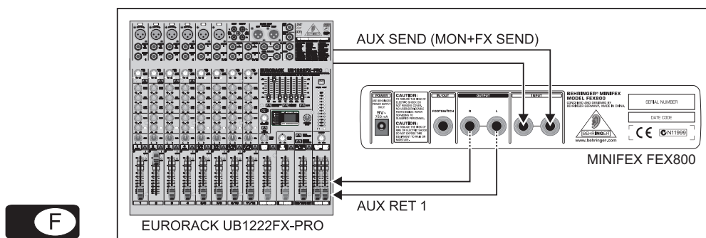
Fig. 4.1 : Câblage du MINIFEX en auxiliaire
