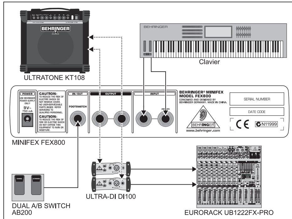
Fig. 4.3 : Câblage du MINIFEX avec un ampli ou des boîtes de direct
