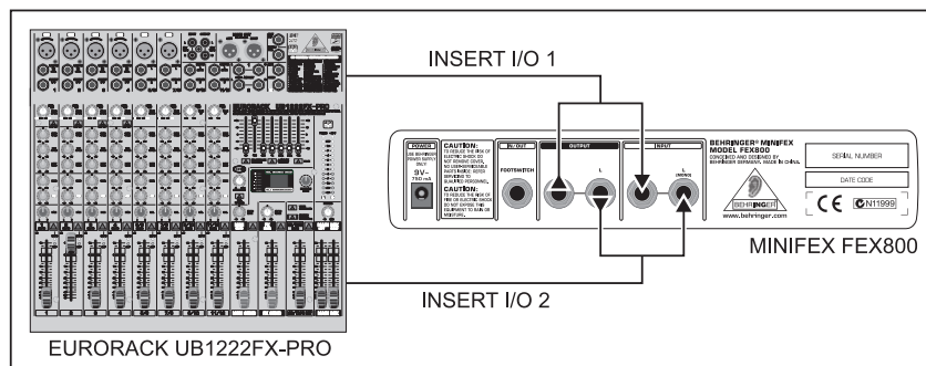
Fig. 4.2 : Câblage du MINIFEX en insert
