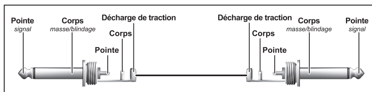
Fig. 5.2 : Liaison asymétrique sur jacks mono
