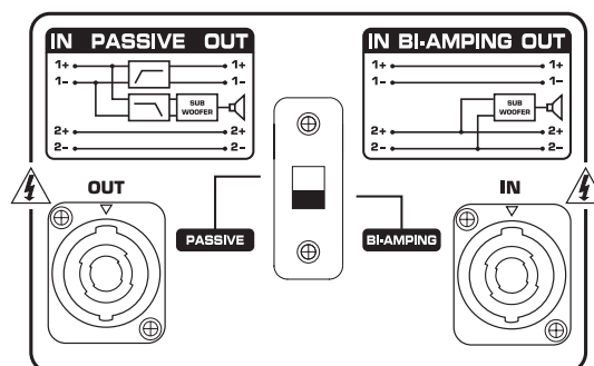
Fig. 1.3 : Connexions des subwoofers
