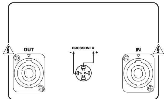
Fig. 1.2 : Connexions des enceintes multivoies Enceinte B1020
