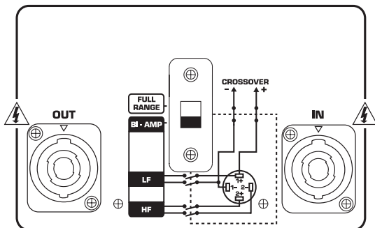
Fig. 1.1 : Connexions des enceintes multi-voies (sauf B1020)
