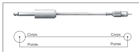
Fig. 9.3: Câble sur jack et Cinch/RCA
