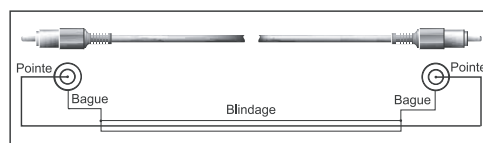
Fig. 9.2: Câble hi-fi sur cinch/RCA
