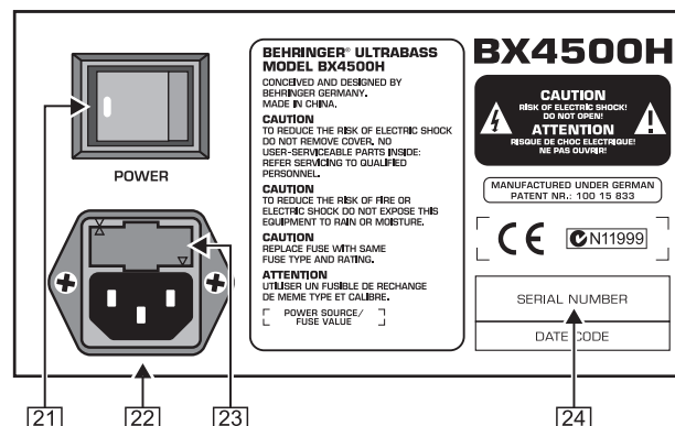
Fig. 2.4 : Panneau arrière du BX4500H (1 ère partie)
