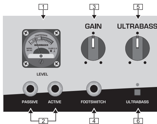
Fig. 2.1 : Face avant du BX4500H (1 ère partie)
