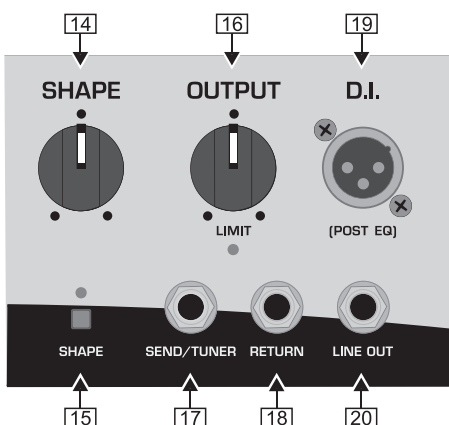
Fig. 2.3 : Face avant du BX4500H (3 ème partie)
