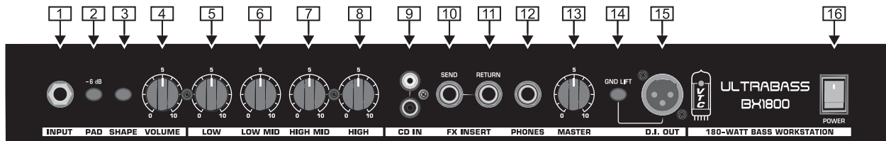
Fig. 3.1 : Commandes et connexions de la face avant
