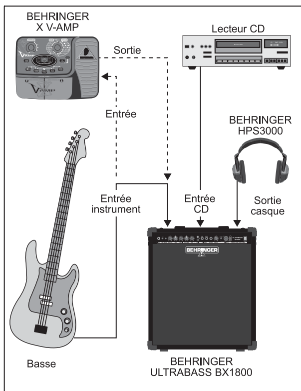
Fig. 2.1 : Exemple d'application avec l'ULTRABASS BX1800
