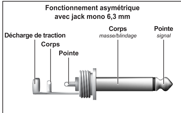
Fig. 4.1 : Jack asymétrique pour l'entrée INPUT
