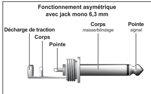
Fig. 4.2 : Jack mono 6,3 mm
