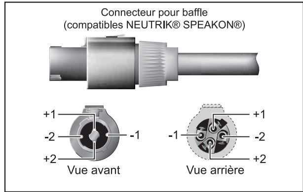
Fig. 4.1 : Connecteur pour baffle professionnel
