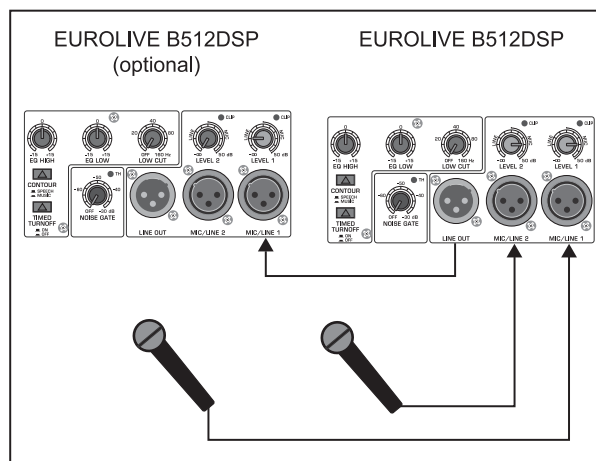
Fig. 3.1 : Câblage de micros
