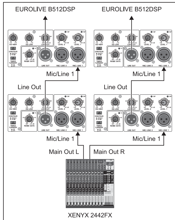
Fig. 3.3 : Chaînage de plusieurs B512DSP
