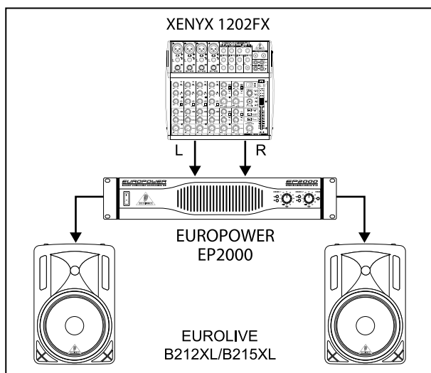
Fig. 5.1 : Utilisation en large bande stéréo
