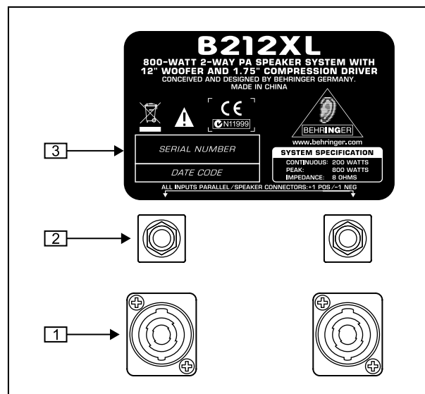
Fig. 2.1 : Connexions (B212XL et B215XL))
