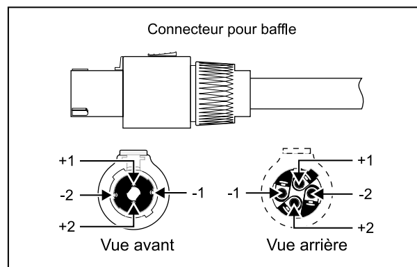
Fig. 6.1 : Connecteur pour baffle
