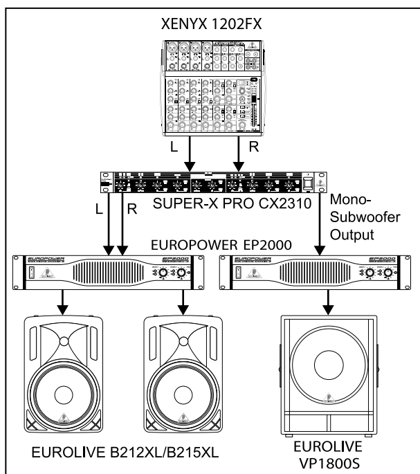
Fig. 5.3 : Utilisation en stéréo avec subwoofer
