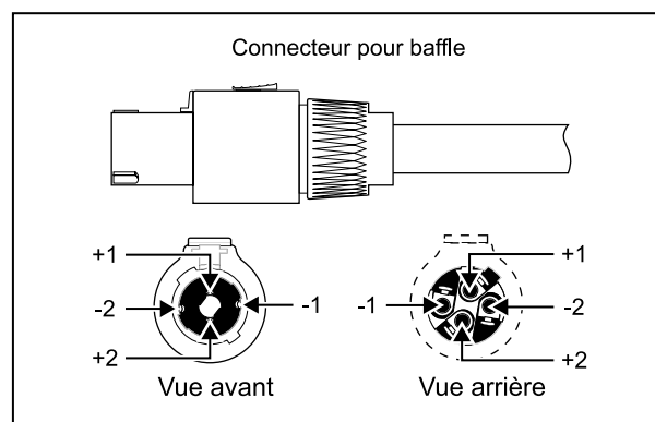
Fig. 6.2 : Jack mono de 6,3 mm
