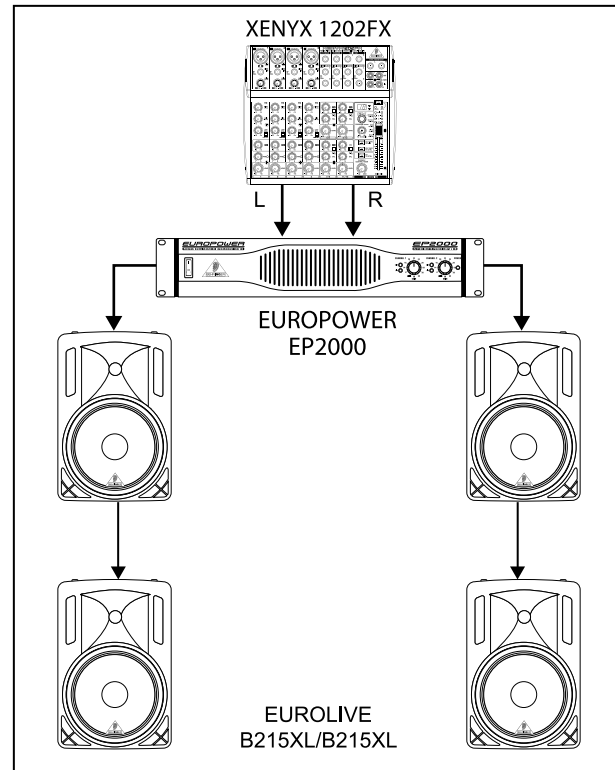
Fig. 5.2 : Câblage de plusieurs B212XL/B215XL
