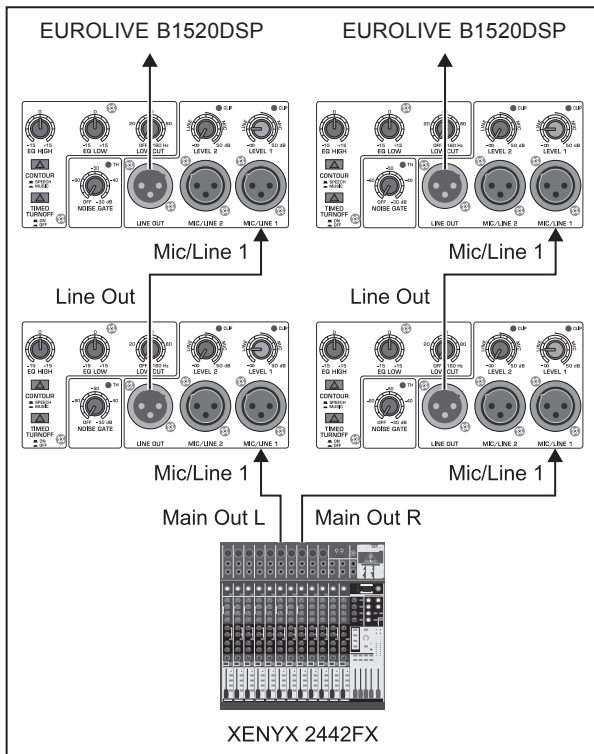
Fig. 3.3 : Chaînage de plusieurs B1520DSP
