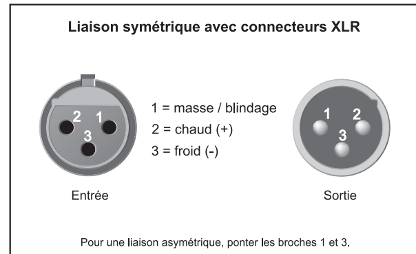
Fig. 4.1 : Connecteurs XLR
