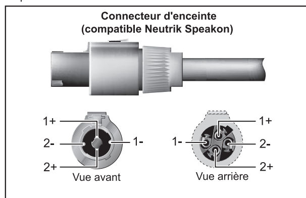
Fig. 1.3: Connecteur Speakon
