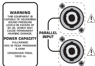
Fig. 1.1: Panneau de connexion des B2520 PRO, B1520 PRO et B1220 PRO
