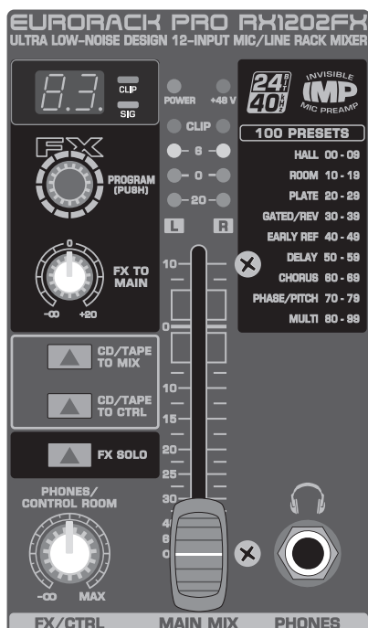
Fig. 2.4 : Commandes de la section Main
