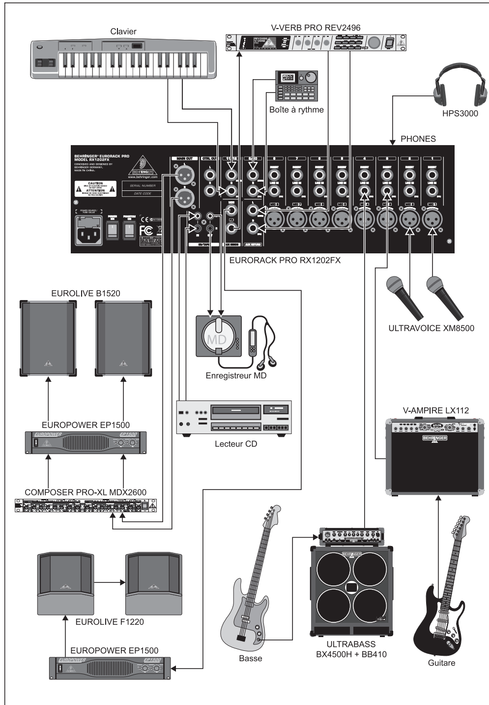
Fig. 3.2 : Application de sonorisation
