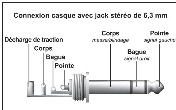
Fig. 4.4 : Jack stéréo pour casque
