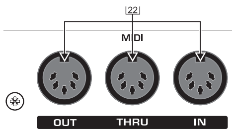
Fig. 3.5 : Connecteurs MIDI du FBQ2496
