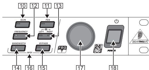
Fig. 3.3 : Partie droite de la face avant du FBQ2496
