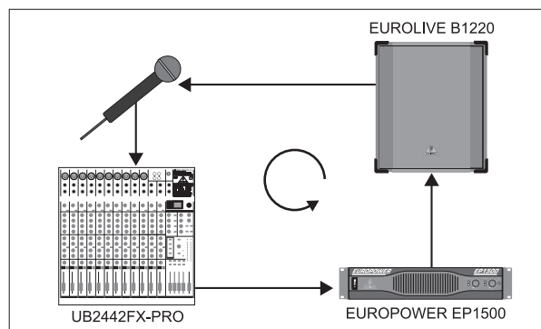
Fig. 2.1 : Formation d'un larsen
