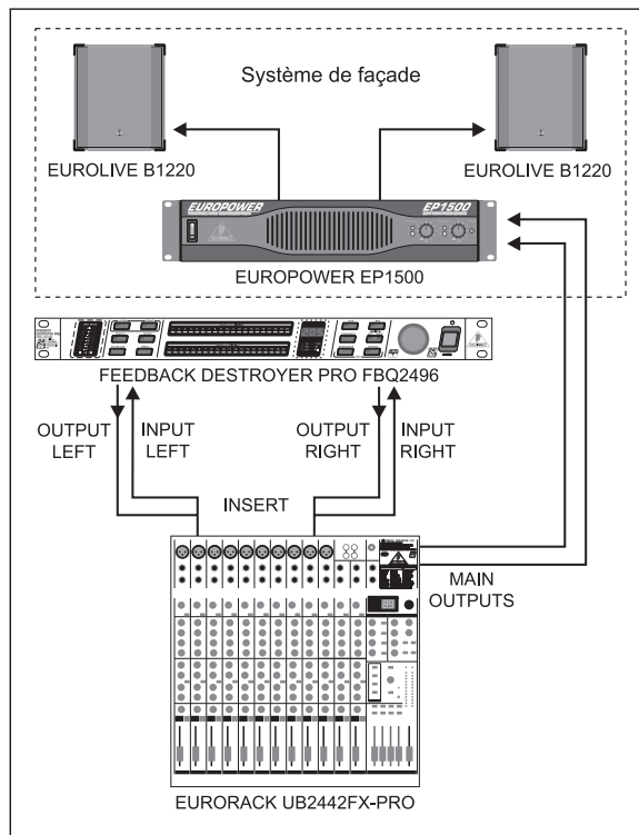
Fig. 5.2 : Le FEEDBACK DESTROYER PRO en insert dans les canaux et les sous-groupes
