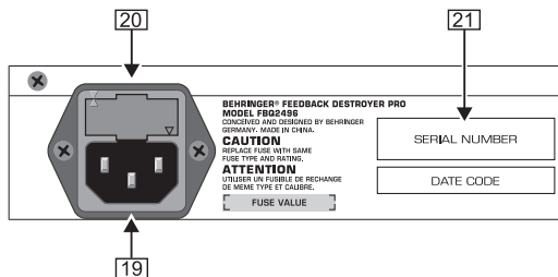
Fig.3.4 : Connexion secteur, porte-fusible et numéro de série
