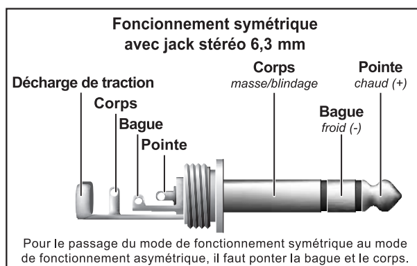
Fig. 8.1 : Jack stéréo de 6,3 mm
