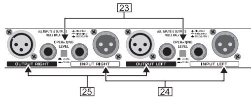
Fig. 3.6 : Connecteurs du panneau arrière du FBQ2496
