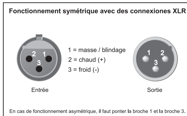
Fig. 8.2 : Connecteur XLR
