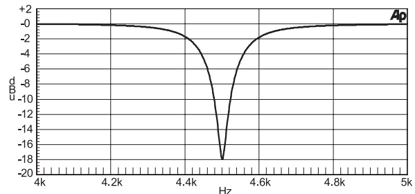
Fig. 4.1 : Courbe d'un filtre très étroit
