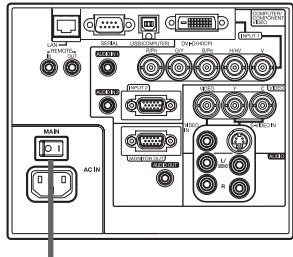
Alimentation principale
