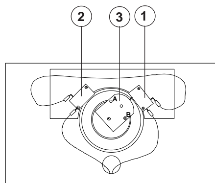
3 - Blocchetto d'azionamento microinterruttori Microswitch tripping block Bloc d'actionnement des microinterruteurs Mikroschalter-Betätigungsblock Bloque accionamiento microinterrutores
