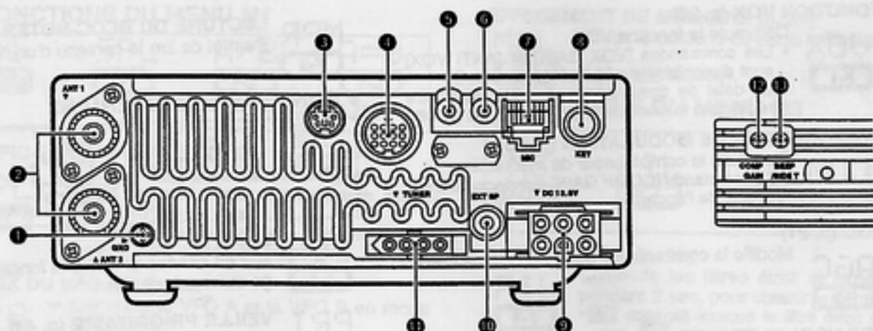
Branchement d'un manipulateur à simple contact ("pioche")
