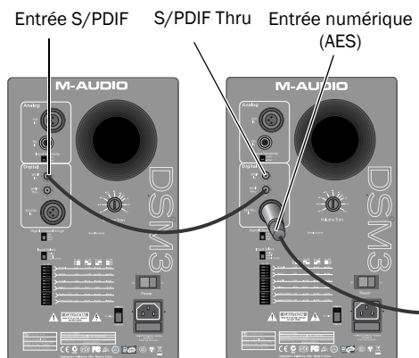
Connexions In et Thru pour l'entrée numérique (source AES)
