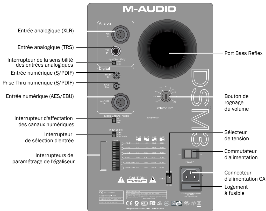
Figure 1. Panneau arrière du haut-parleur DSM3
