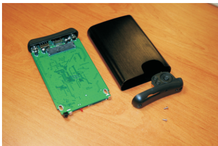
4. Retournez la carte mère afin d'accéder à l'emplacement du disque dur.
