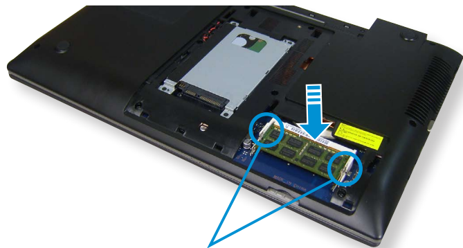
Loquets du module de mémoire
