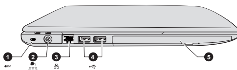
Illustration 3-2 Ordinateur vu de gauche
