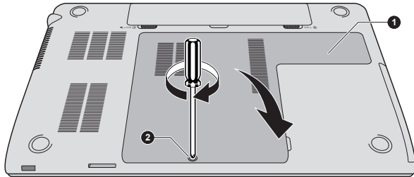
Illustration 4-15 Retrait du capot du module mémoire
