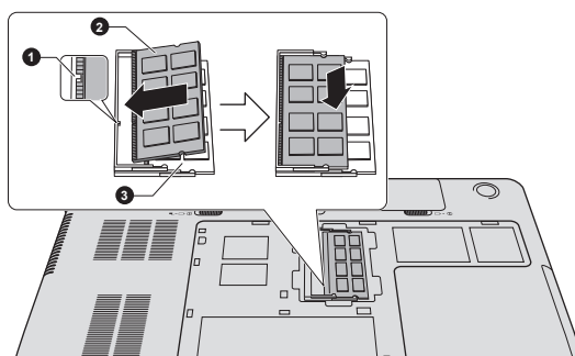
Illustration 4-14 Pose du module mémoire
