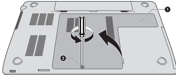
Illustration 4-13 Retrait du couvercle du module mémoire
