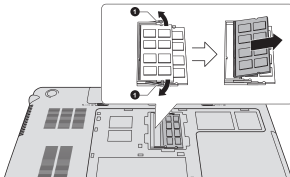
Illustration 4-16 Retrait d'un module mémoire
